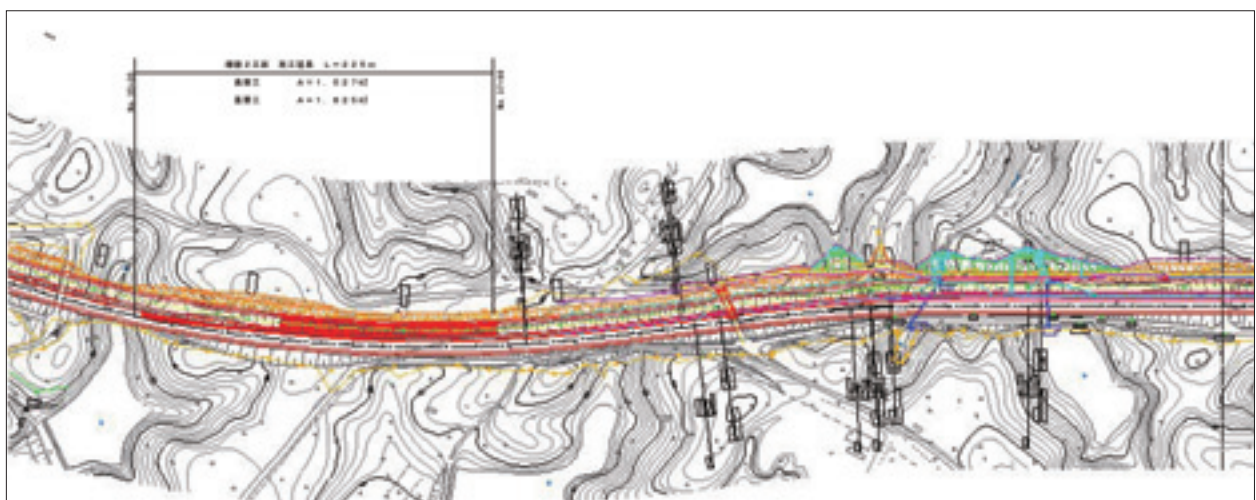
平面図
