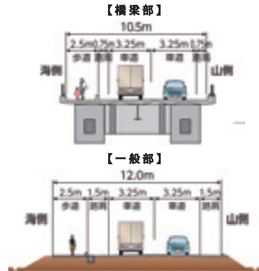
図-2 標準断面図
