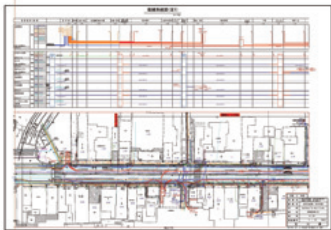
管路配管系統図
