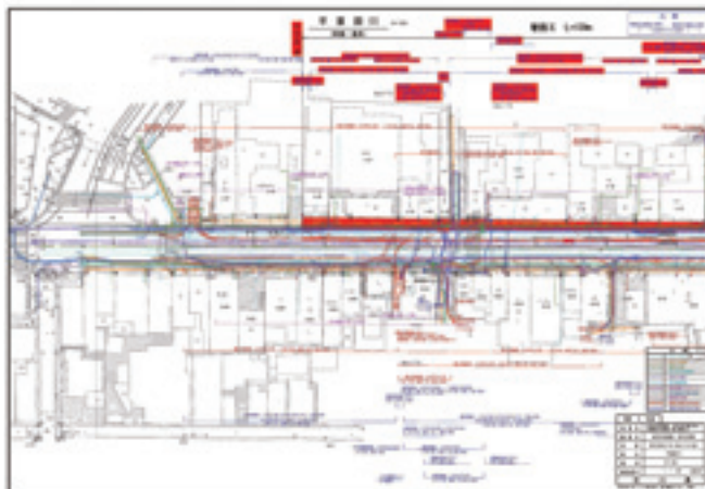
埋設管平面図
