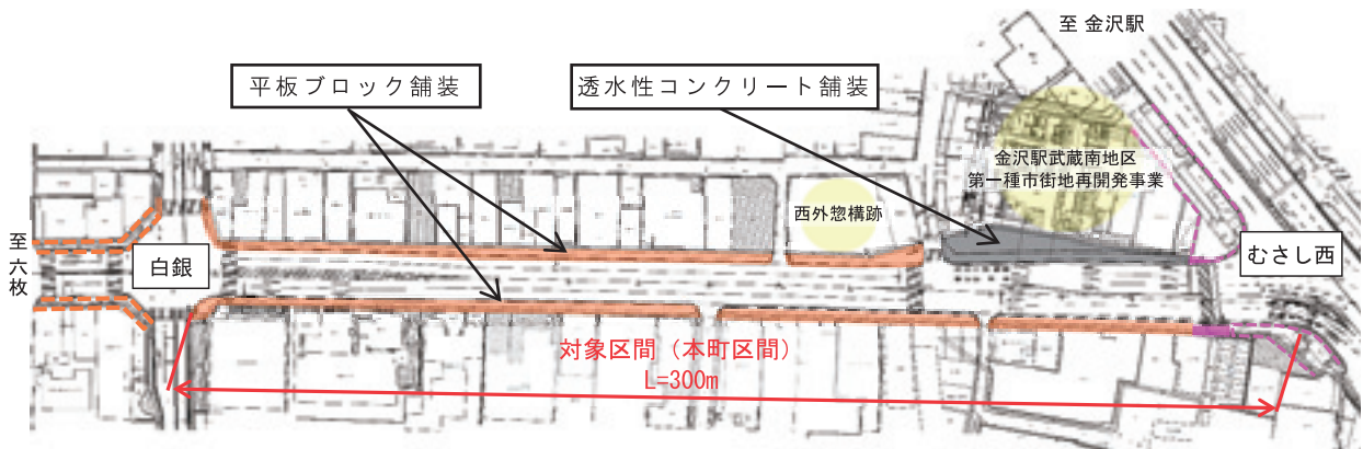
図-3 歩道舗装図面
