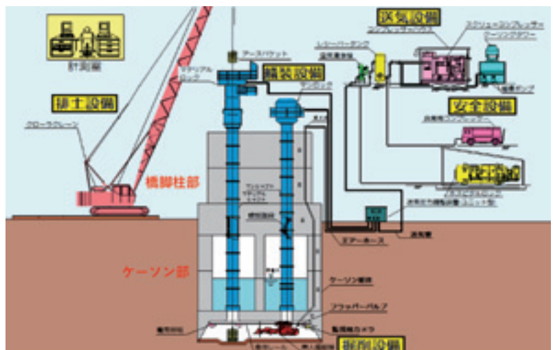
ケーソン設備の概要図
