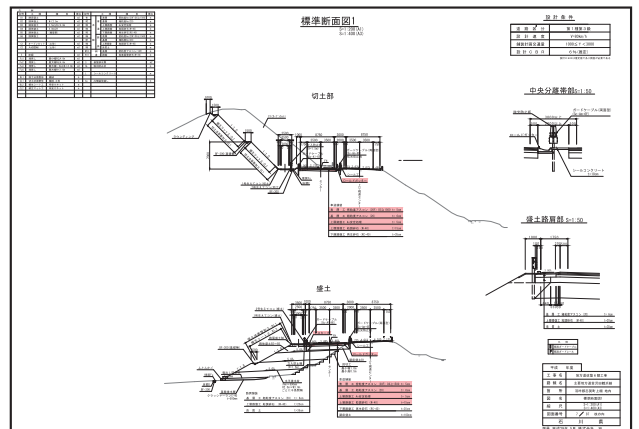
標準断面図1
