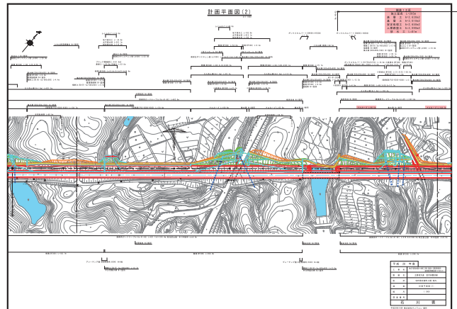
計画平面図(2)
