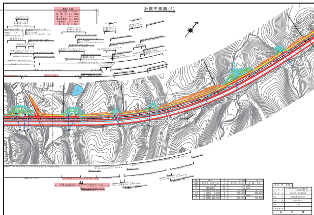
計画平面図(3)
