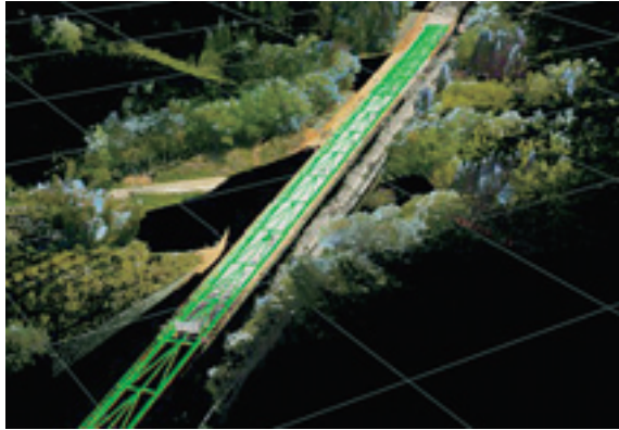
起工測量の結果と3次元元設計データの照合確認
